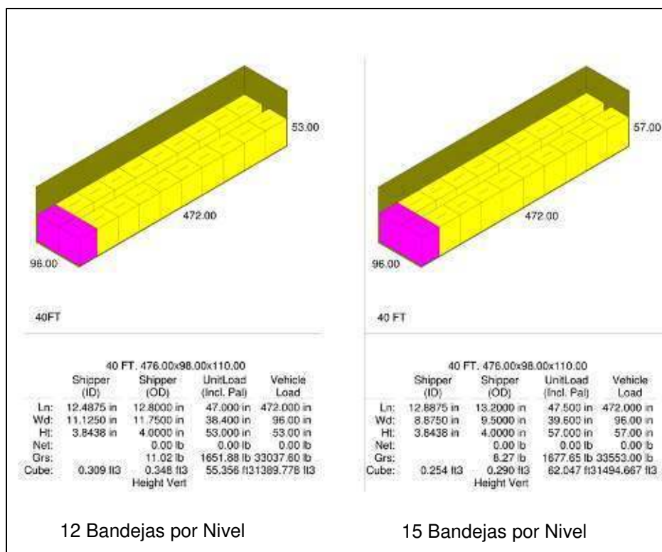
Figura 12: Carga de bandejas de mango paletizadas en un contenedor de 40 pies
