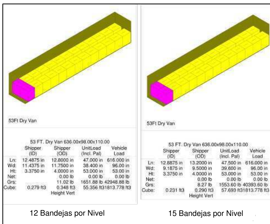
Figura 13: Carga de bandejas de mango paletizadas en un contenedor de 53 pies
