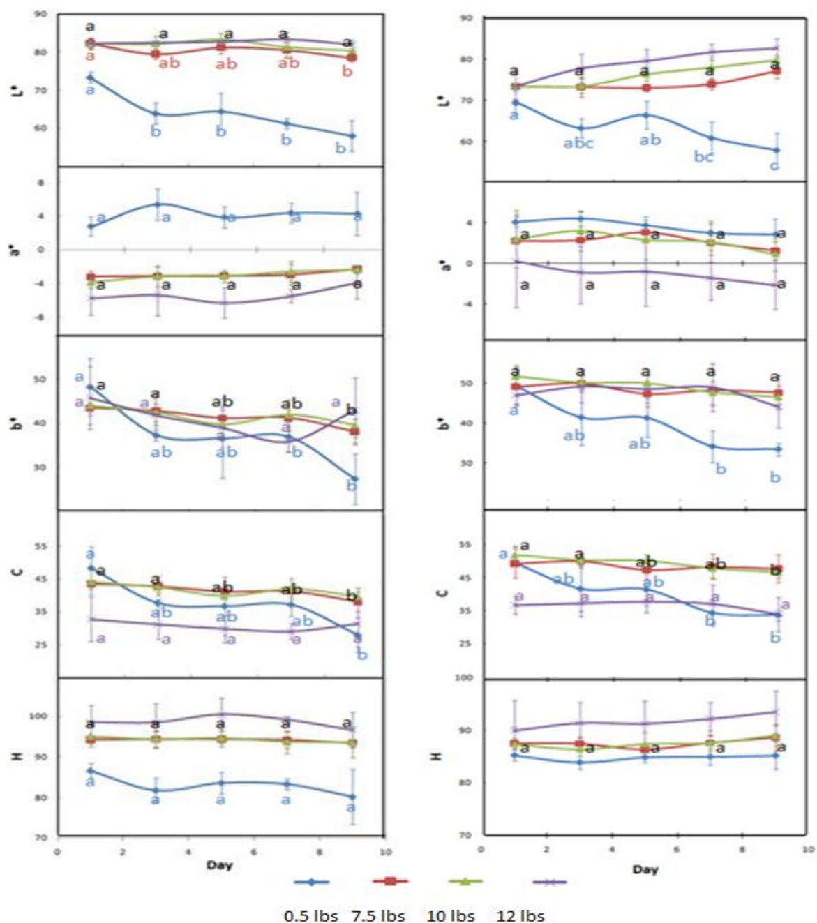
Figura 9. Cambios en L^* (luminosidad), a^* (verde / rojo), b^* (azul / de color amarillo), C (croma o saturación de color y ángulo hue ( H ) en los cubos de mango provenientes de mangos enteros con diferentes firmeza de la pulpa exterior al momento del corte. Las rebanadas fueron tomados del lado exterior (a la izquierda) y del lado interior (derecha) y se almacenaron a 5^\circ\text{C} durante 9 días.
